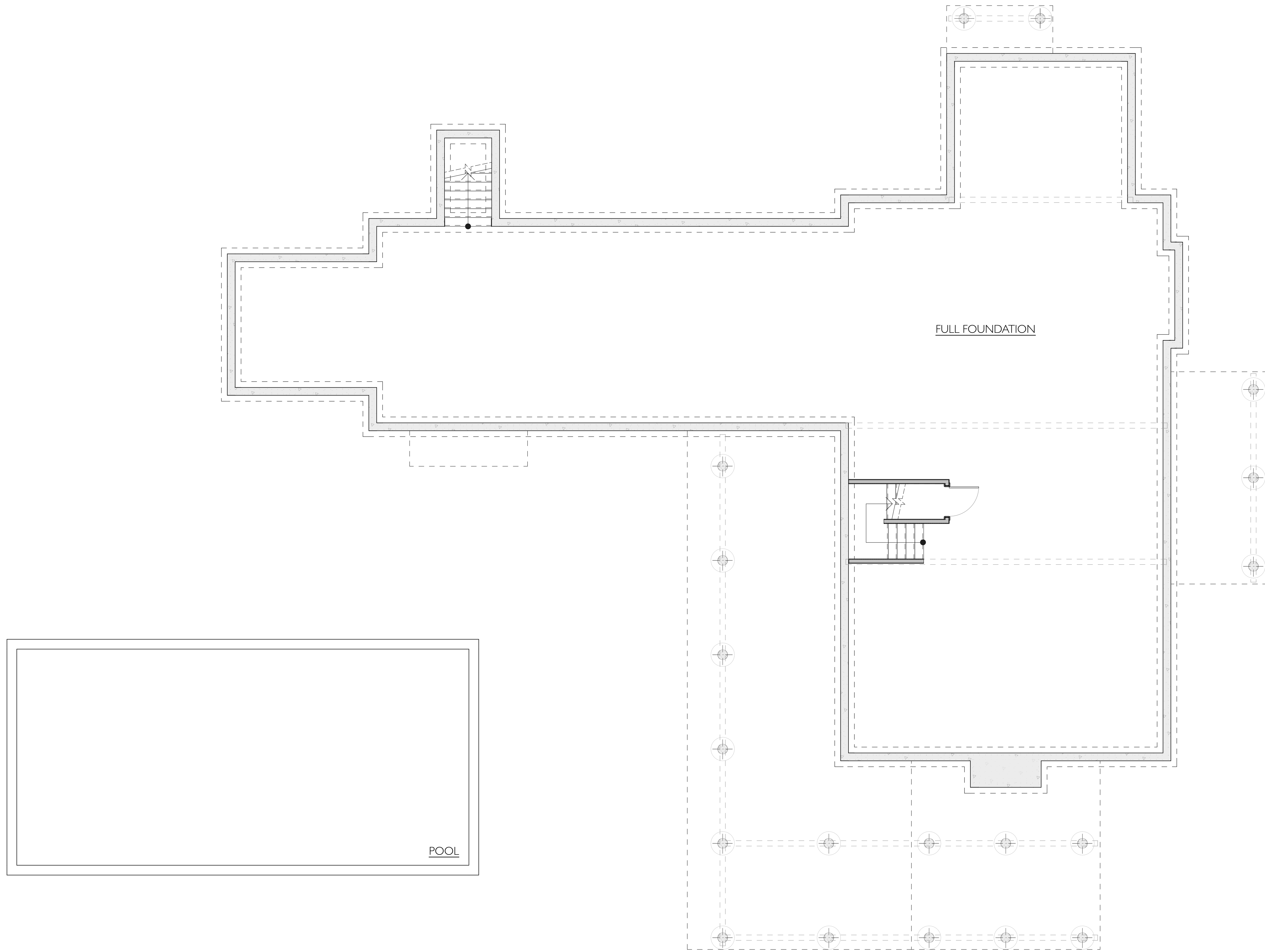
FOUDATION PLAN
